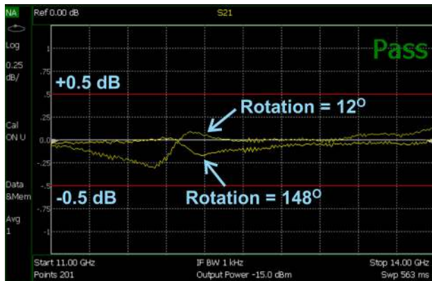
(a) S21 Log Mag
